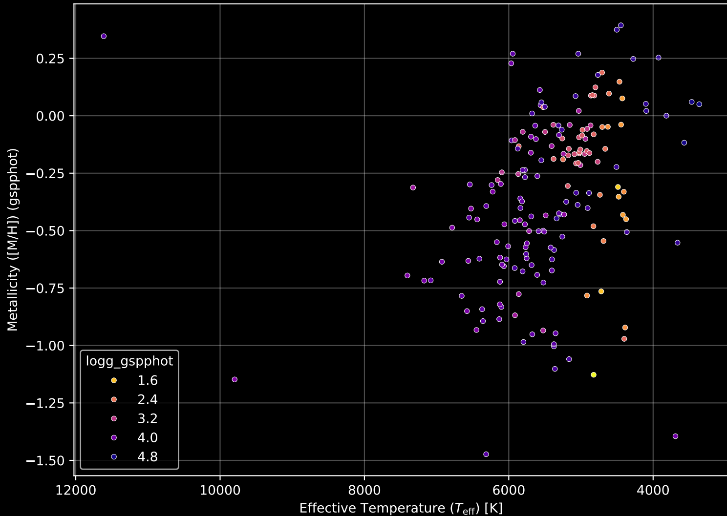
APOGEE DR17 Field: [290-28-O_TESS] Stellar Population Parameters (n= 180)
